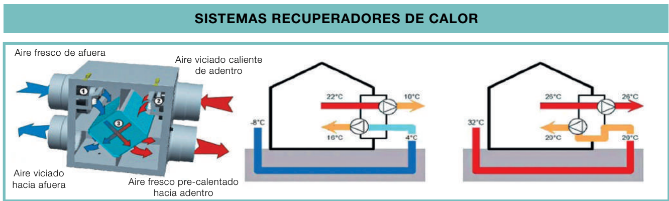
Figura 14. Sistemas recuperadores de calor
