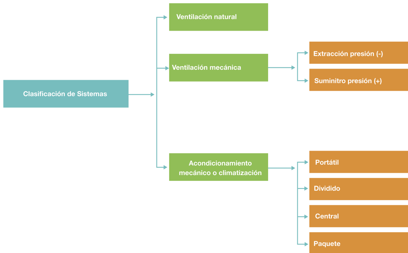
Figura 7. Clasificación de los sistemas de ventilación, climatización o acondicionamiento de aire
